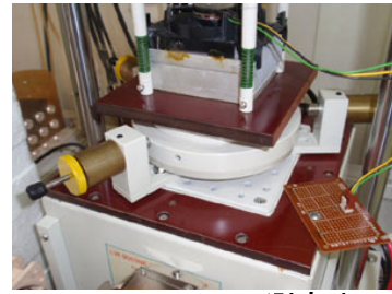
ASTM D5470 測定中
