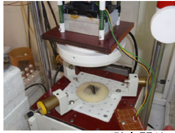
ASTM D5470 測定開始
