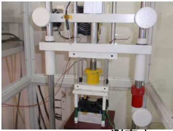
ASTM D5470測定中
