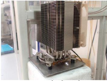
インテル方式測定
