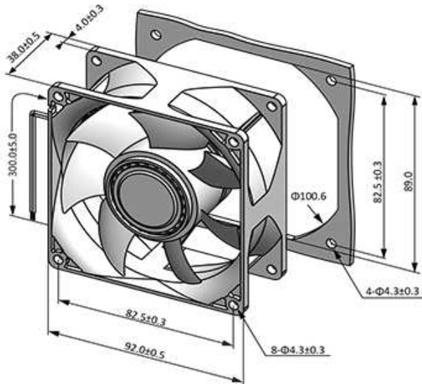
■ Dimensions (Unit:mm)
