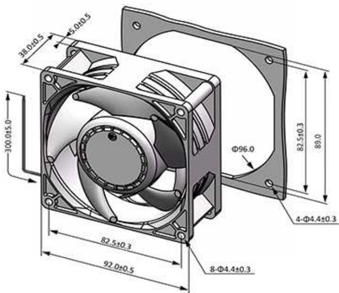
■ Dimensions (Unit:mm)
