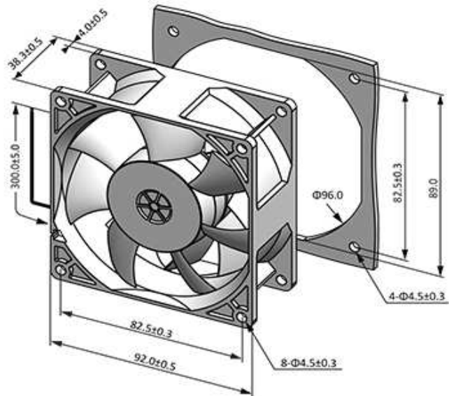
■ Dimensions (Unit:mm)
