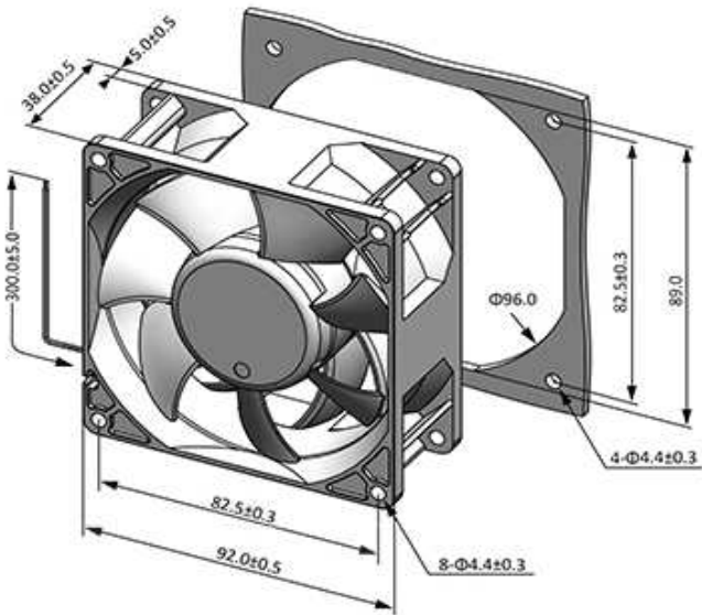
■ Dimensions (Unit:mm)
