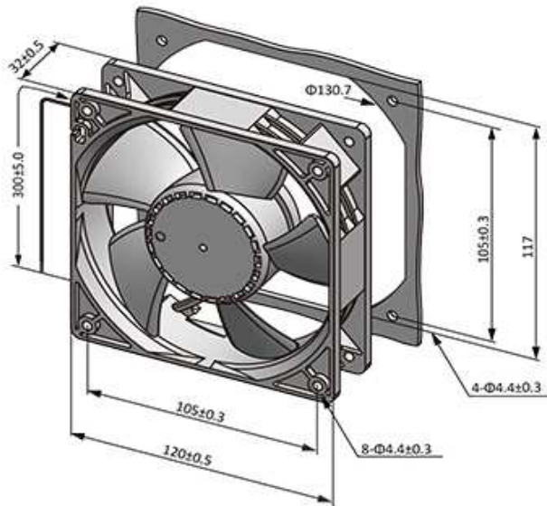
■ Dimensions (Unit:mm)
