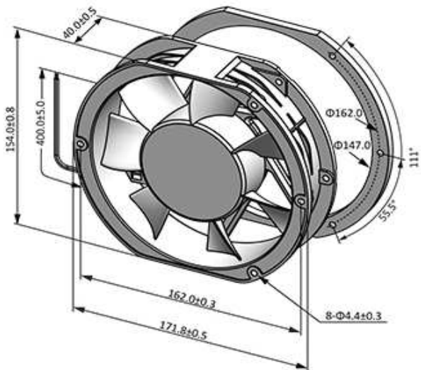
■ Dimensions (Unit:mm)
