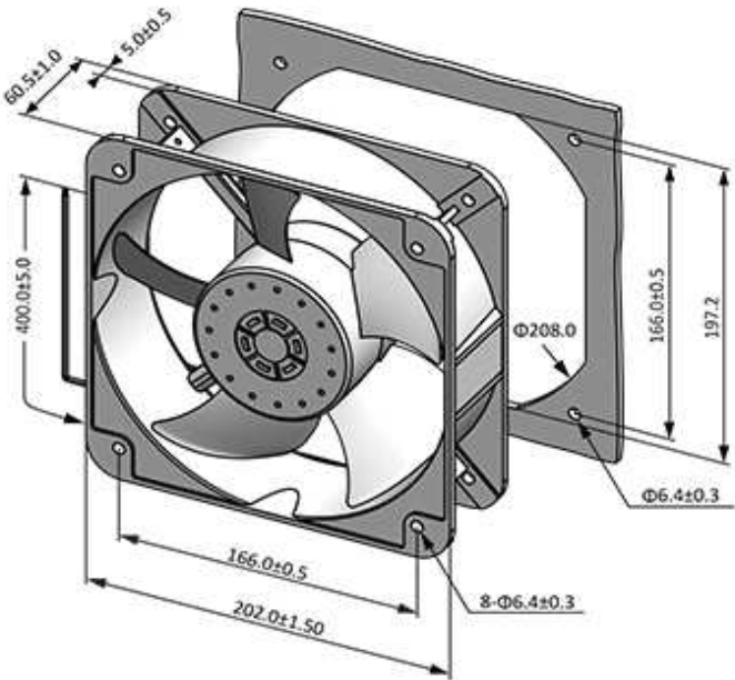
■ Dimensions (Unit:mm)
