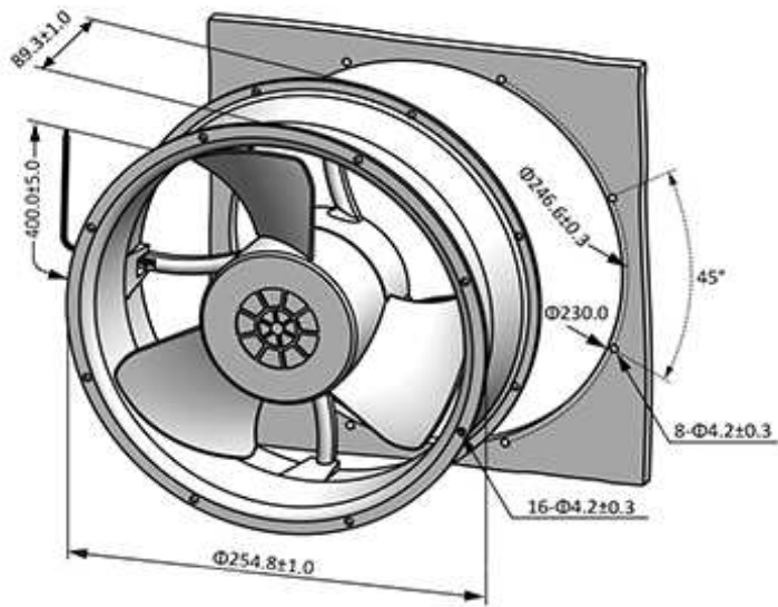
■ Dimensions (Unit:mm)
