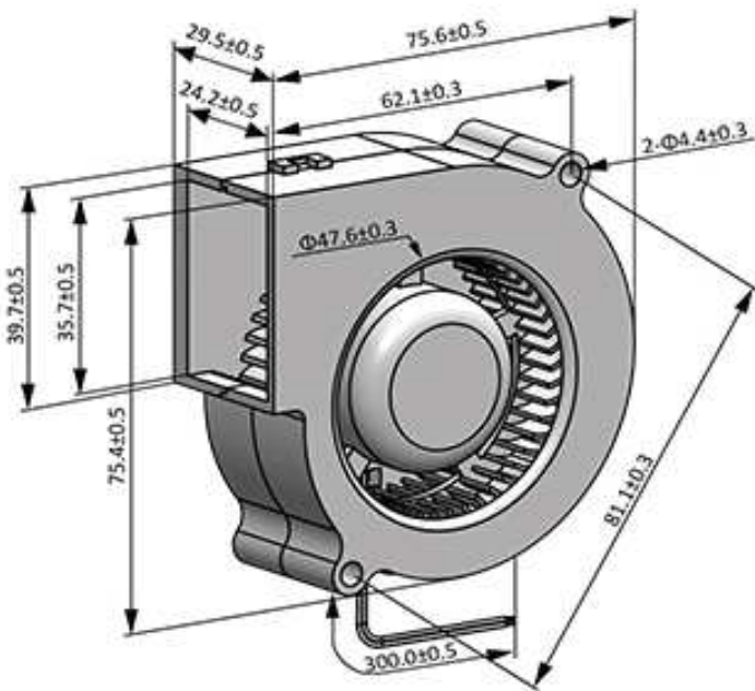
■ Dimensions (Unit:mm)
